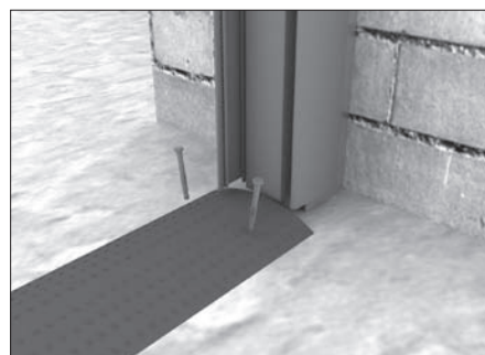
Просверлите 4 отверстия \varnothing 13 в дорожном покрытии и в «лежащем полицейском». Вбейте анкерные болты. Затяните гайки на анкерных болтах.
